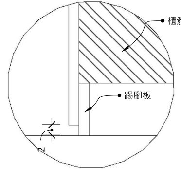
詳圖C: 衣櫃門片施工大樣 比例: 1/5
